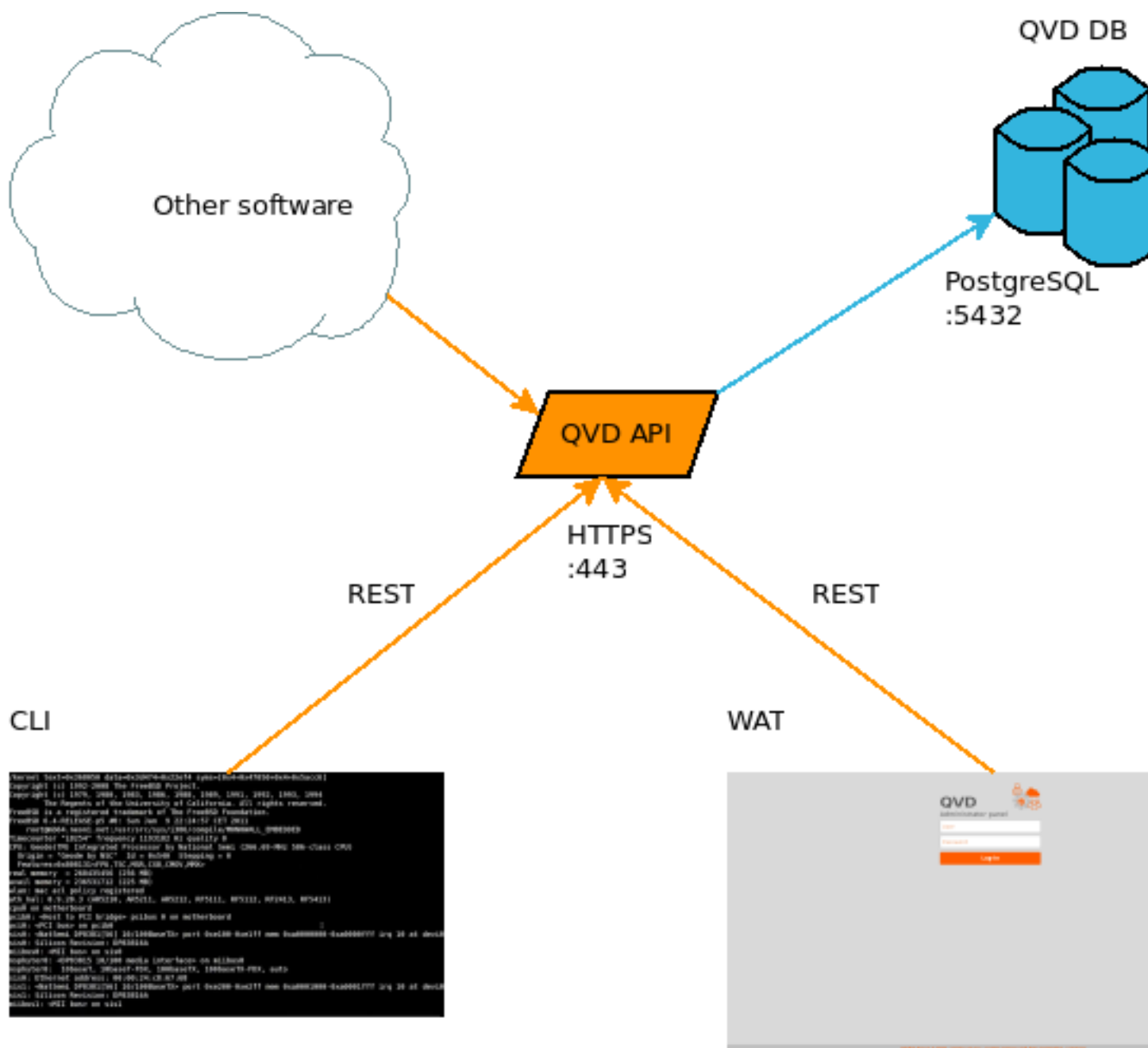
Figure 2: Componentes de un nodo de Administración
